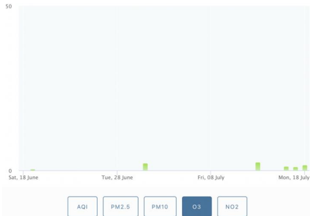
Gambar 6. Hasil pengukuran O 3 Jakarta
