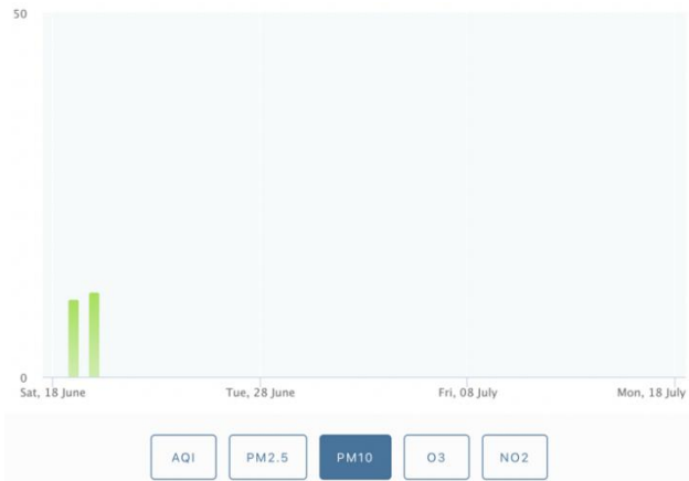
Gambar 5. Hasil pengukuran PM 10 Jakarta
